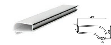
5 MM TEK CAM ÇITA PROFİLİ
