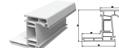
PERVAZLI KASA PROFİLİ
