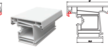
DIŞA AÇILIR KAPI PROFİLİ
