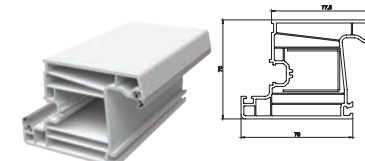
İÇE AÇILIR KAPI PROFİLİ
