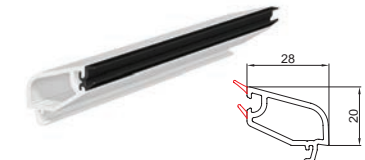
20 MM ÇİFT CAM ÇITA PROFİLİ
